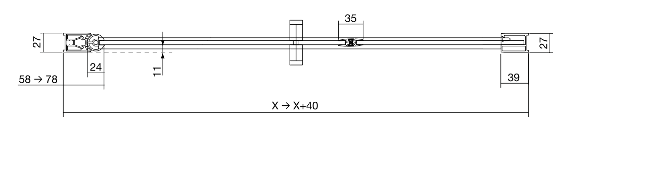
Porta 2 battenti + fisso per angolo (OM2P+OMFX)
