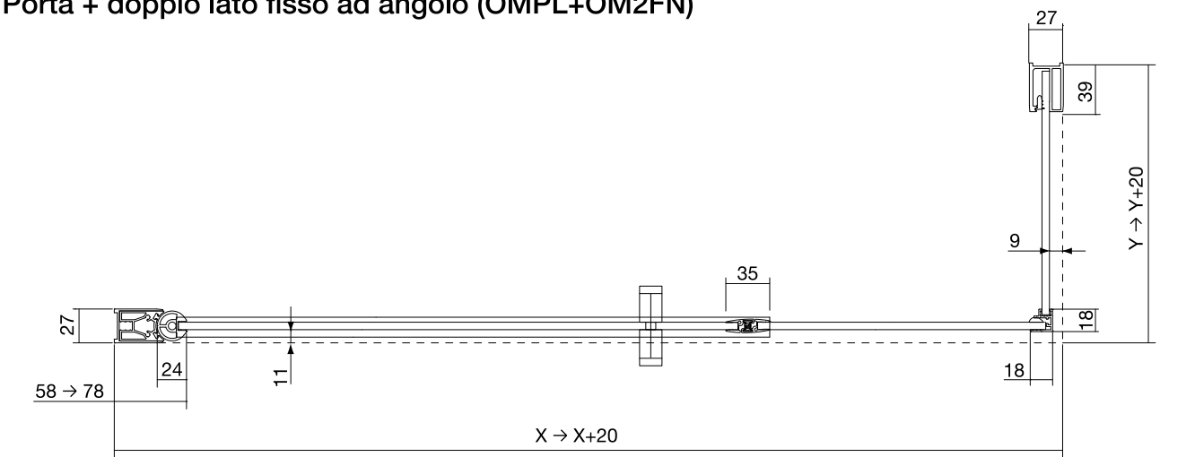
Porta + doppio lato fisso ad angolo (OMPL+OM2FN)
