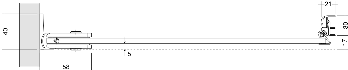
Porta con cerniera muro-vetro per nicchia (art. PRJCMN)
