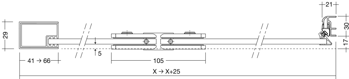
Porta con cerniera vetro-vetro per nicchia (art. PRJCVN)
