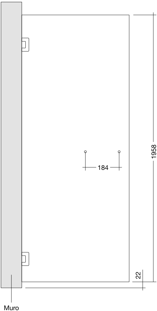
Porta con cerniera muro-vetro
