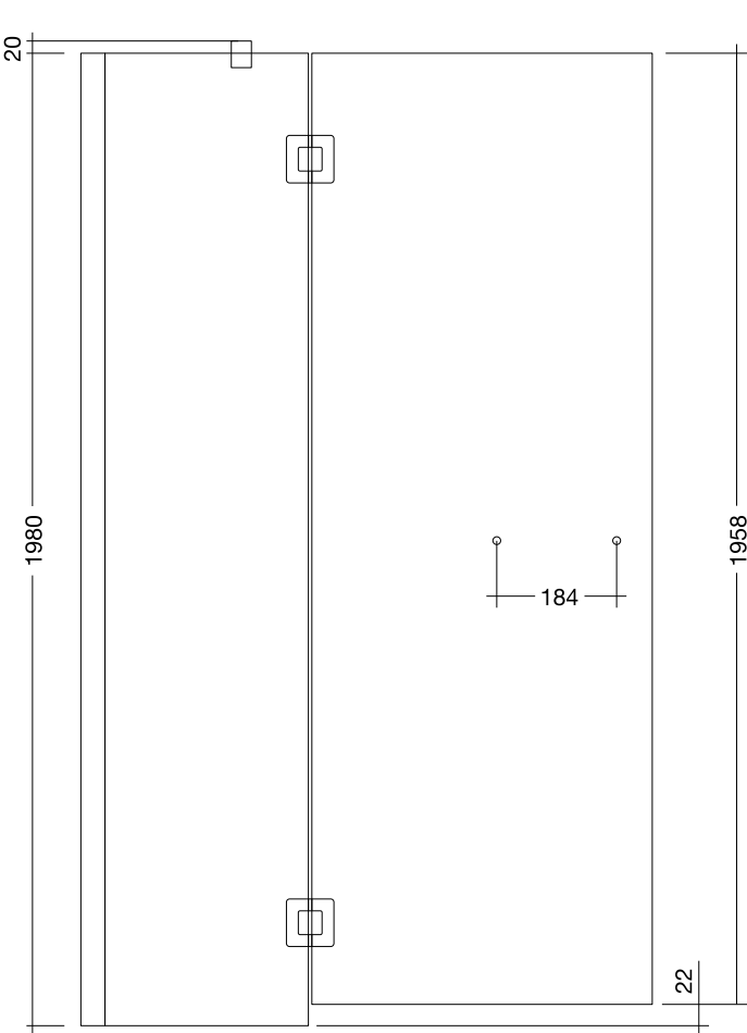
Porta con cerniera vetro-vetro
