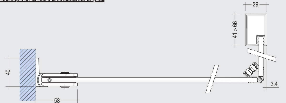
Vista dall'alto porta con cerniera MURO-VETRO ad angolo
