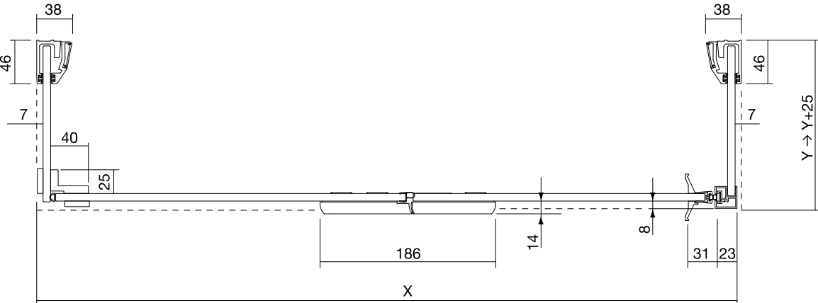
Porta con doppio fisso a parete (art. IVPOX-IVFX)
