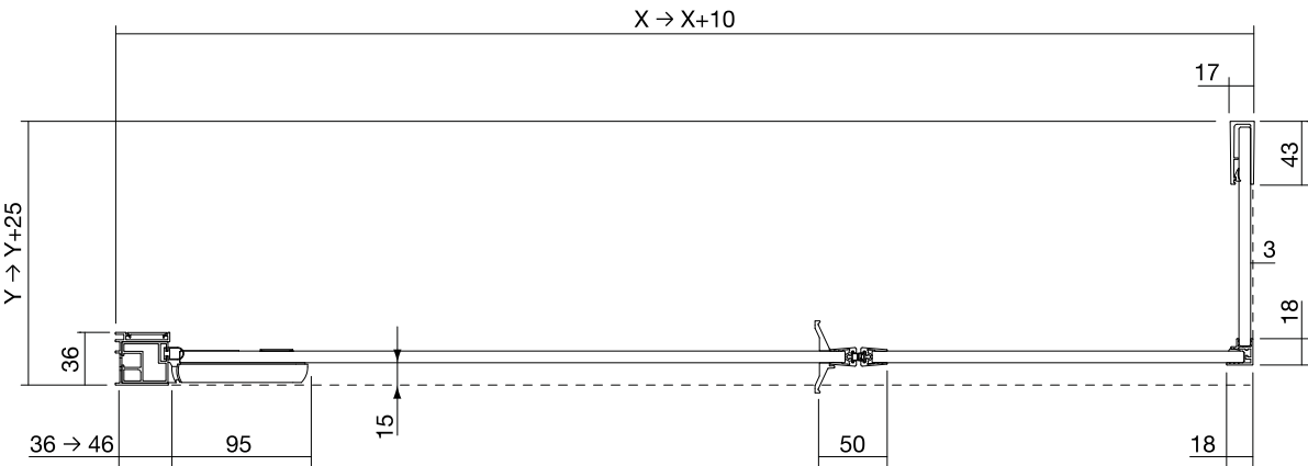
Porta battente + doppio fisso ad angolo (art. IMPL-IM2F)
