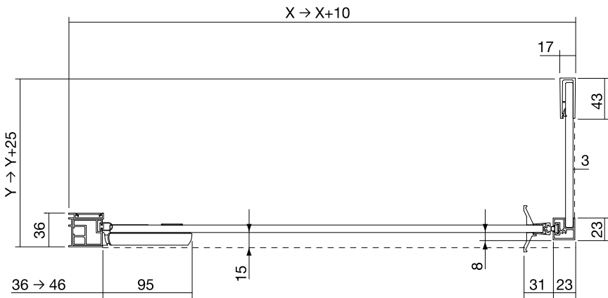
Porta battente + fisso per angolo (art. IMPO-IMFI)
