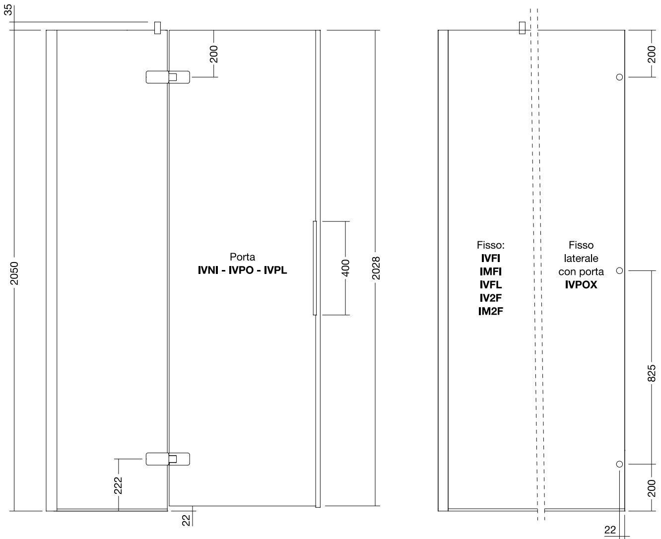
Composizioni particolari - Fisso su muretti
