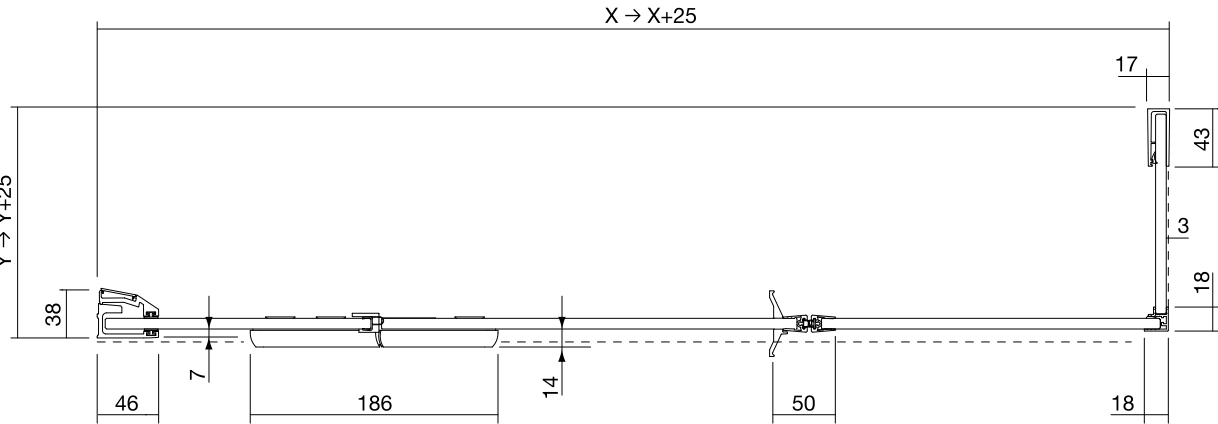
Porta battente + doppio fisso ad angolo (art. IVPL-IV2F)
