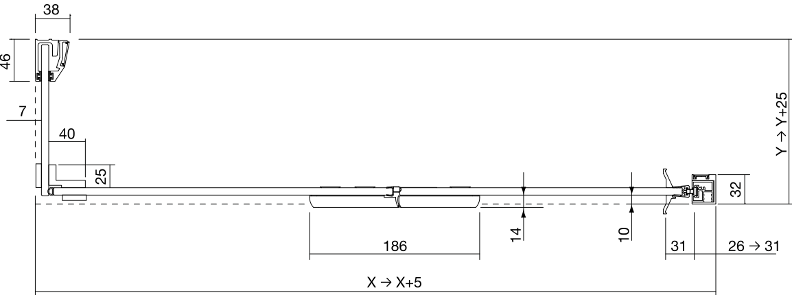
Porta con doppio fisso per angolo (art. IVPOX-00PFBTIO)
