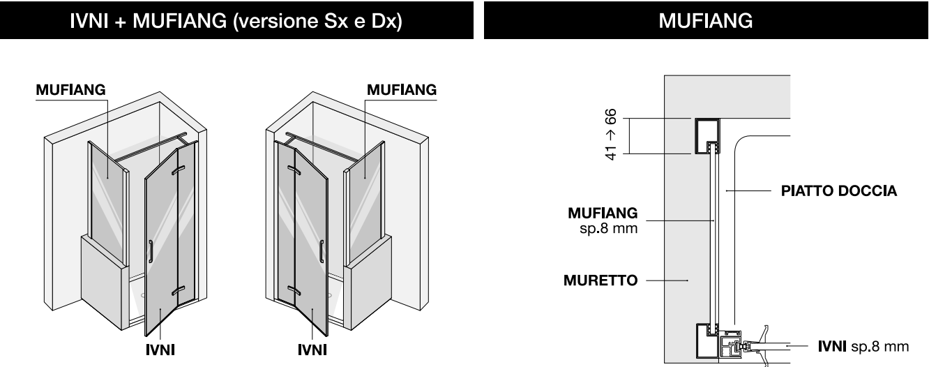
Composizioni particolari - Fisso su muretti
